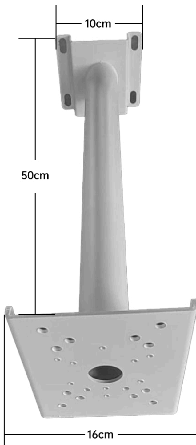
Rysunek referencyjny wymiarów i instalacji produktu
